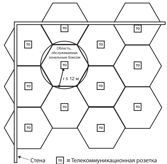
Рисунок 4: Пример построения ячеек для выбора места расположения зональных боксов
